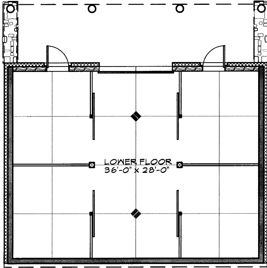
2 LOWER FLOOR PLAN A2 SCALE: 1/8" = 1'-0"
